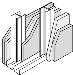
Assonometria
