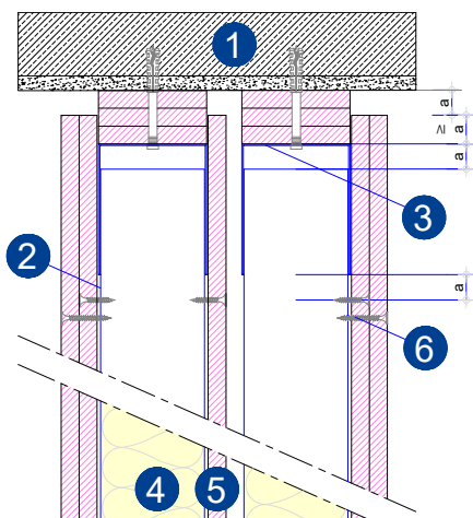
SAD5 CON INTERCAPEDINE CENTRALE
