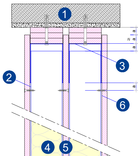
SAD5 CON INTERCAPEDINE CENTRALE
